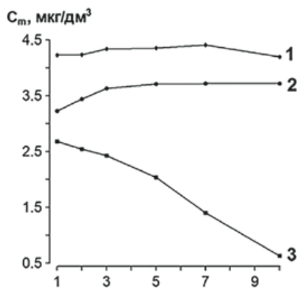
Рис. 4. Зависимость концентрации бромпроизводных нитрофенолов в водном растворе от продолжительности бромирования: 1 – 3-нитрофенол, 2 – 4-нитрофенол, 3 – 2-нитрофенол; C(\text{Br}_2) = 0.001 \text{ моль/дм}^3 , C(\text{KBr}) = 0.1 \text{ моль/дм}^3
