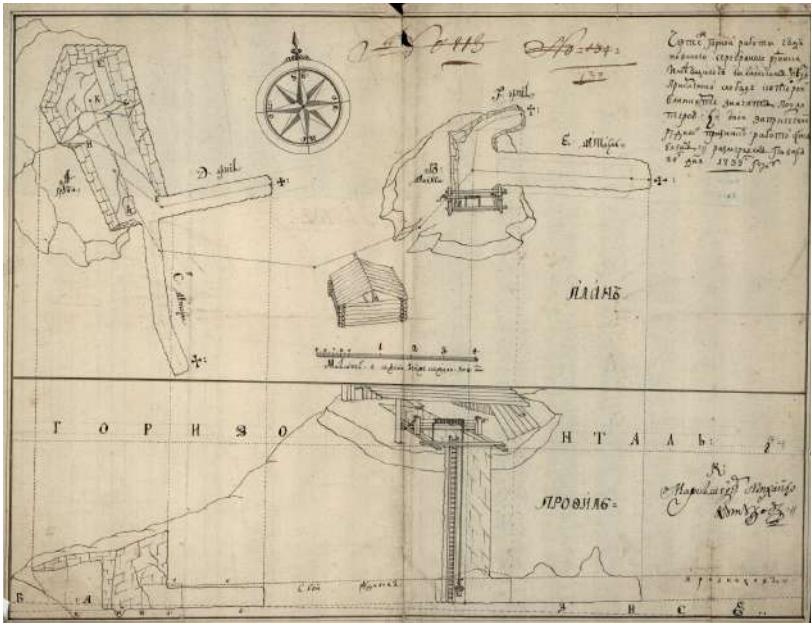
Рис. 3. Чертеж горной работы Чудиновского серебряного рудника. Илимский уезд. 1733 г. Автор: маркшейдер Михайло Кутузов. ГАСО. Ф. 59. Оп. 7. Д. 15. Л. 1.
