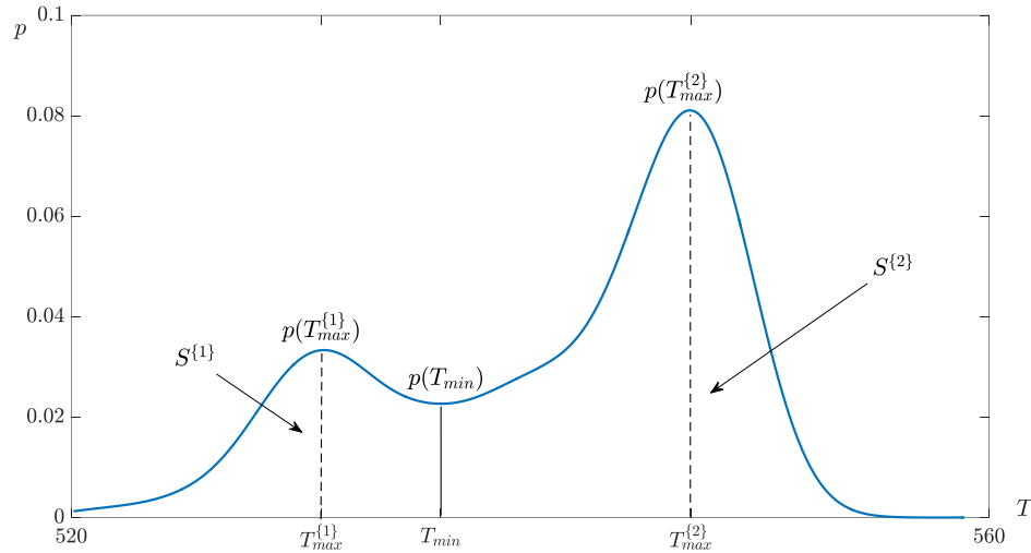
Рис. 6. Аппроксимация РП p(T) ПР ВР \tilde{T}_{3950, \tilde{l}}
