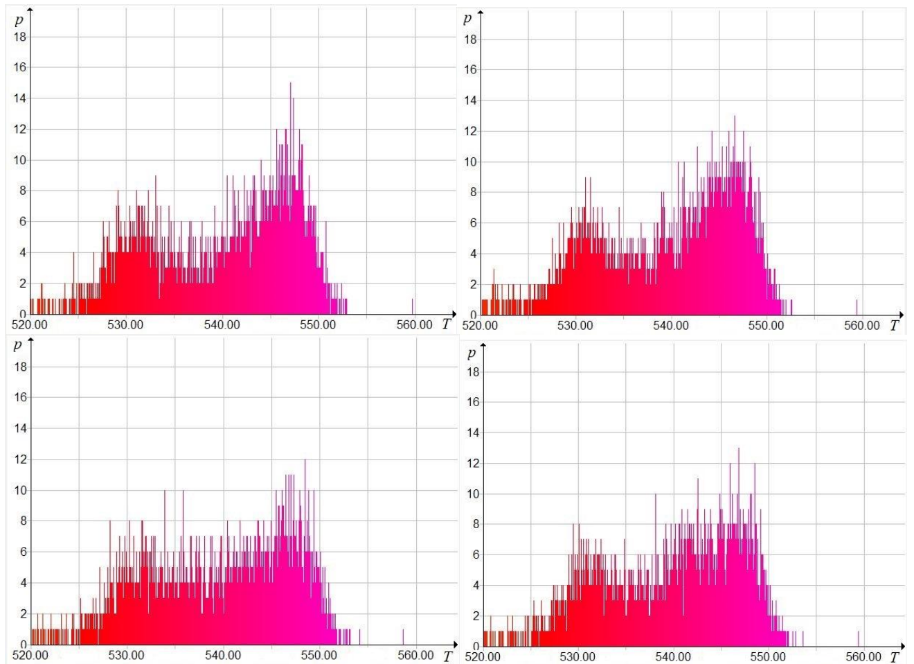
Рис. 5. Гистограммы распределения рядов \tilde{T}_{k=10, \tilde{l}} , \tilde{T}_{k=30, \tilde{l}} , \tilde{T}_{k=40, \tilde{l}}
