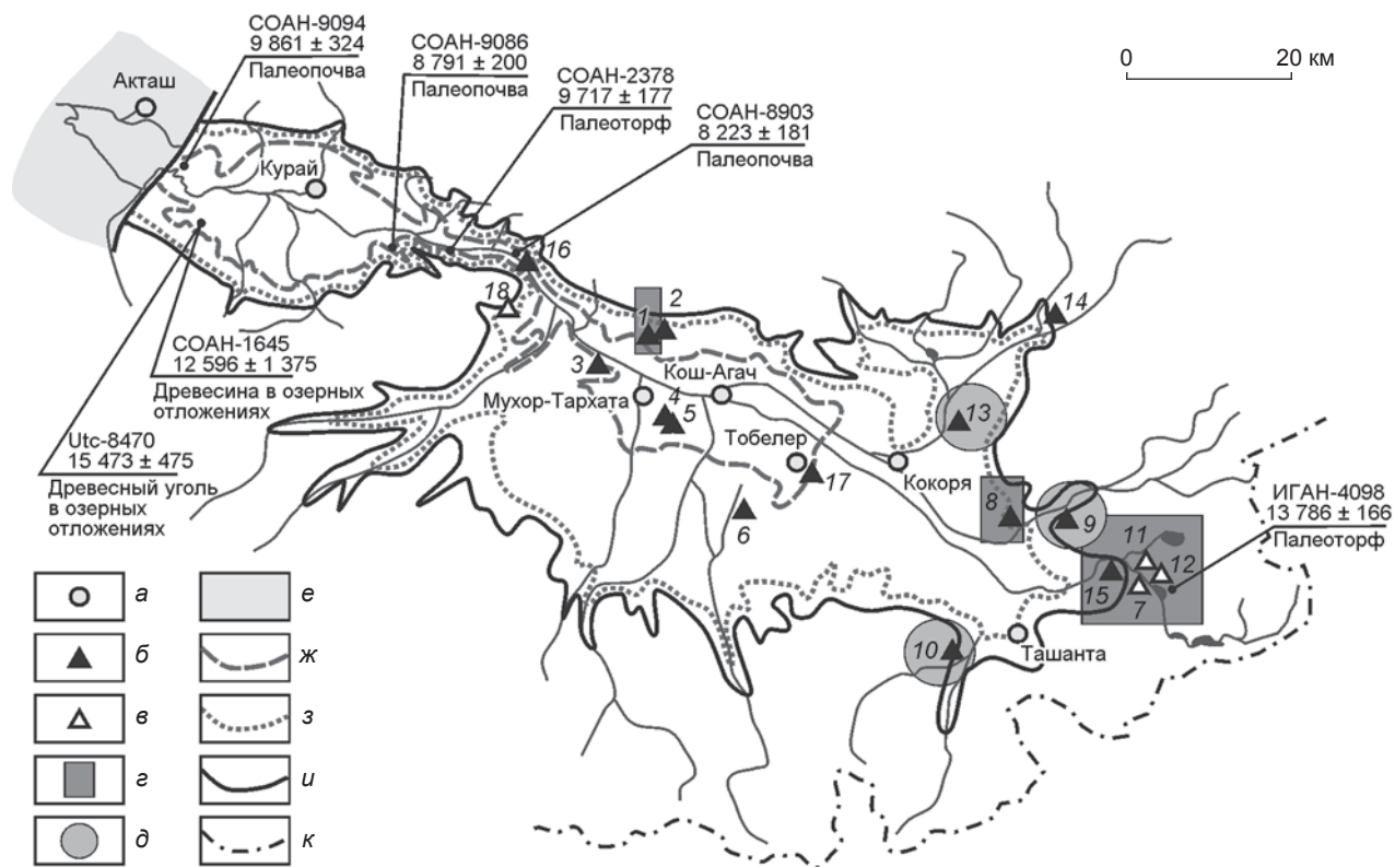
Рис. 1. Соотношение позднепалеолитических памятников с уровнями палеозер в Курайско-Чуйской системе впадин и основные радиоуглеродные даты (калиброваны на 2\sigma ), характеризующие развитие ландшафтов этих впадин в конце позднего неоплейстоцена – раннем голоцене.
