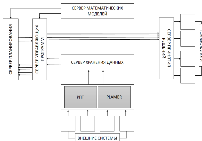
Рис. 7 Комплекс программ «Управление транспортными процессами в условиях противоречивости»
