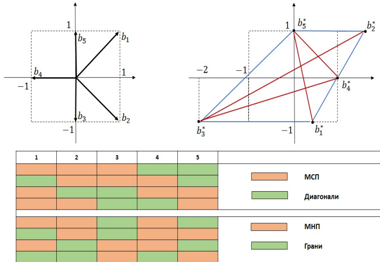
Рис. 1 Комбинаторные свойства многогранников и несовместных систем линейных неравенств
