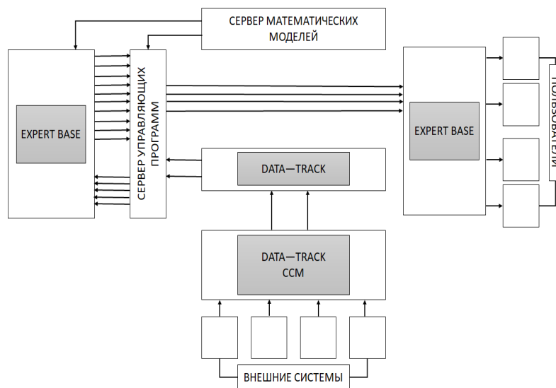
Рис. 6 Комплекс программ «Управление технологическими маршрутами на дискретном производстве»
