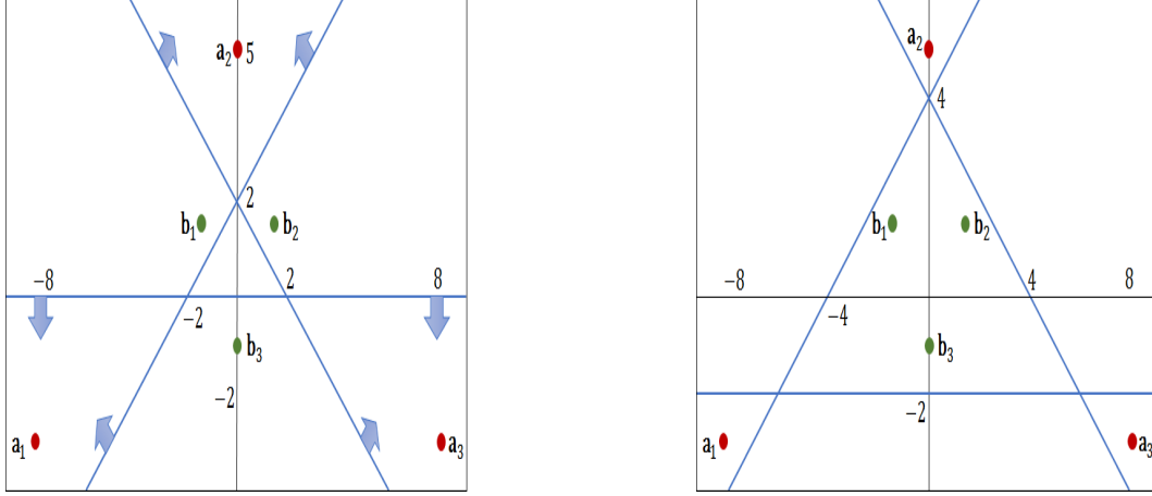
Рис. 2 Комитеты и альтернативные покрытия
