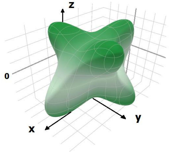
Рисунок 2 – Зависимость модуля Юнга от направления в кристалле \text{Lu}_2\text{Si}_2\text{O}_7 , построенное по рассчитанным в данной работе значениям упругих модулей.
