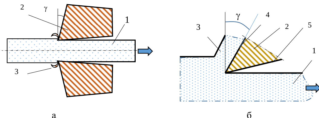
Рисунок 11 – Схема скальпирования прутковой заготовки (а) и увеличенное изображение места съема стружки (б): 1 – заготовка; 2 – скальпирующая волока; 3 – стружка, 4 и 5 – передняя и задняя кромки резца соответственно, стрелка показывает направление перемещения заготовки
