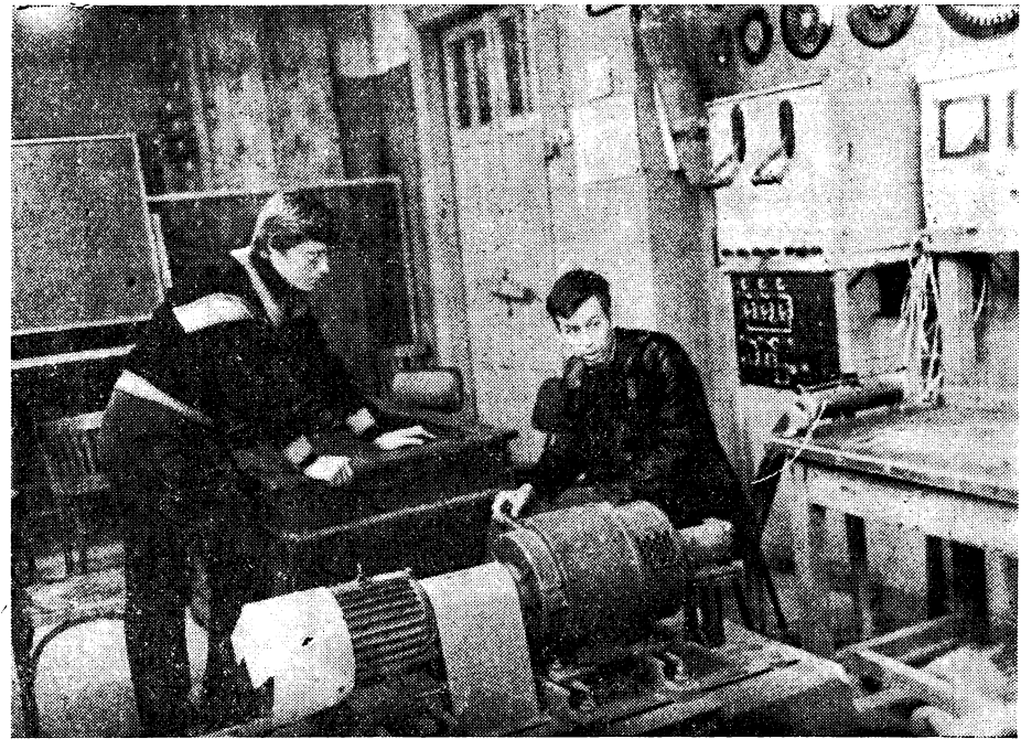
На снимке: И. Е. РОДИОНОВ, доцент, кандидат технических наук, руководитель темы по разработке синхронного частотно-регулируемого двигателя для электромобиля, и С. Г. Хайнин, сотрудник проблемной лаборатории. Фото Г. РЕДОЗУБОВОЙ. Фотохроника УПИ.
