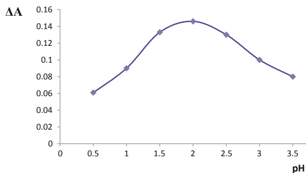
Рис. 4. Зависимость \Delta A кремний-титановых ксерогелей, модифицированных пирокатехиновым фиолетовым, от pH. Время контакта 10 минут, \lambda = 560 нм. \Delta A = A_0 - A_{200} , где A_0 и A_{200} – оптические плотности модифицированных кремний-титановых ксерогелей в отсутствие фторид-ионов и в присутствии 200 мг/л фторид-ионов, соответственно
