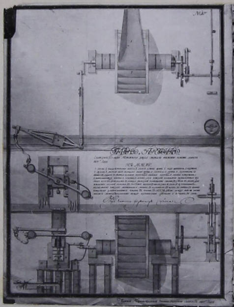
Стан для тиснения монеты.
