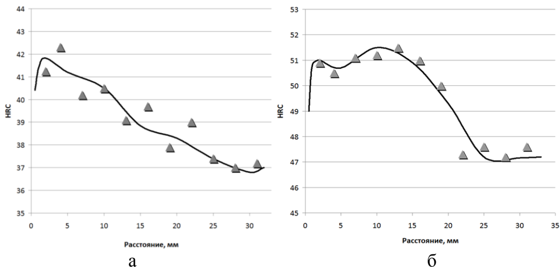
Рис. 2. Распределение твердости по сечению заготовки диаметром 100 мм из стали 25Г2С2Н2МА после охлаждения: а) в потоке воздуха; б) в масле
