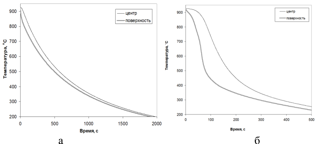
Рис.1. Расчетные траектории охлаждения заготовок диаметром 100 мм из стали 25Г2С2Н2МА: а) в потоке воздуха; б) в масле
