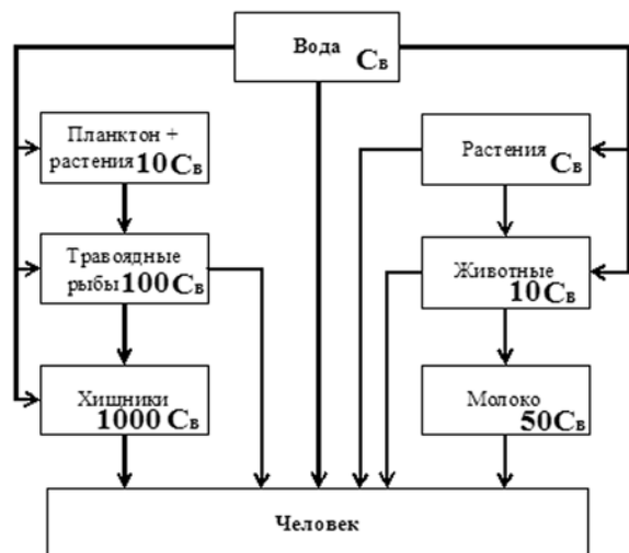
Рис. 2. Модель распределения вещества в экосистеме с учетом сделанных предположений
