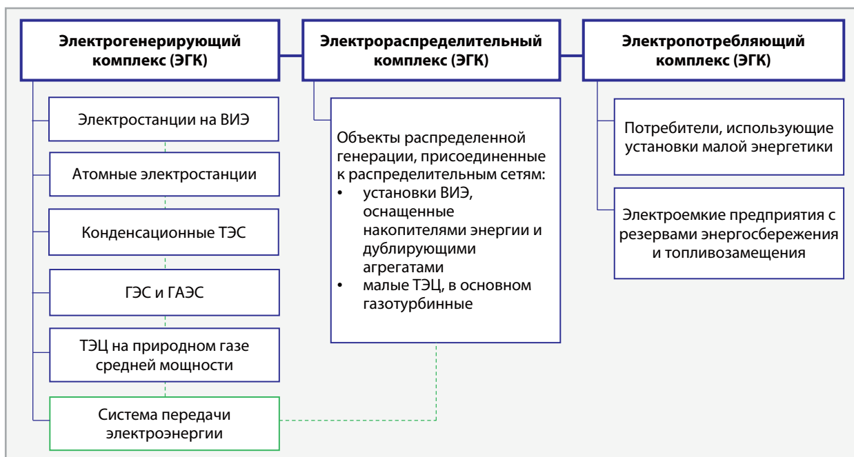
Рис. 3. Структура идеальной модели региональной электроэнергетики (источник: разработано авторами)
