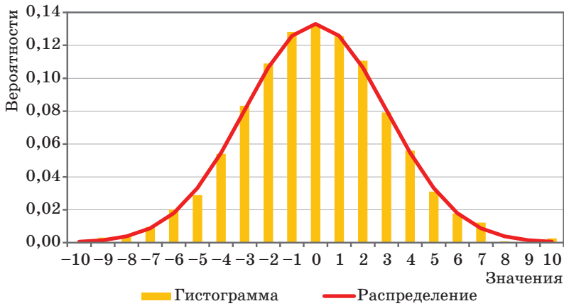
Рис. 2. Гистограмма нормального распределения \mu = 0 ; \sigma = 3
