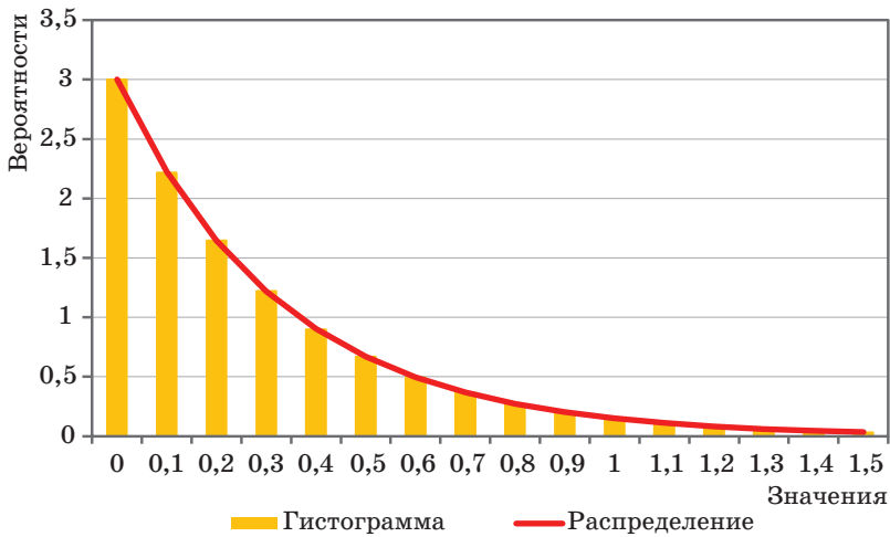
Рис. 3. Гистограмма экспоненциального распределения \sigma = 3
