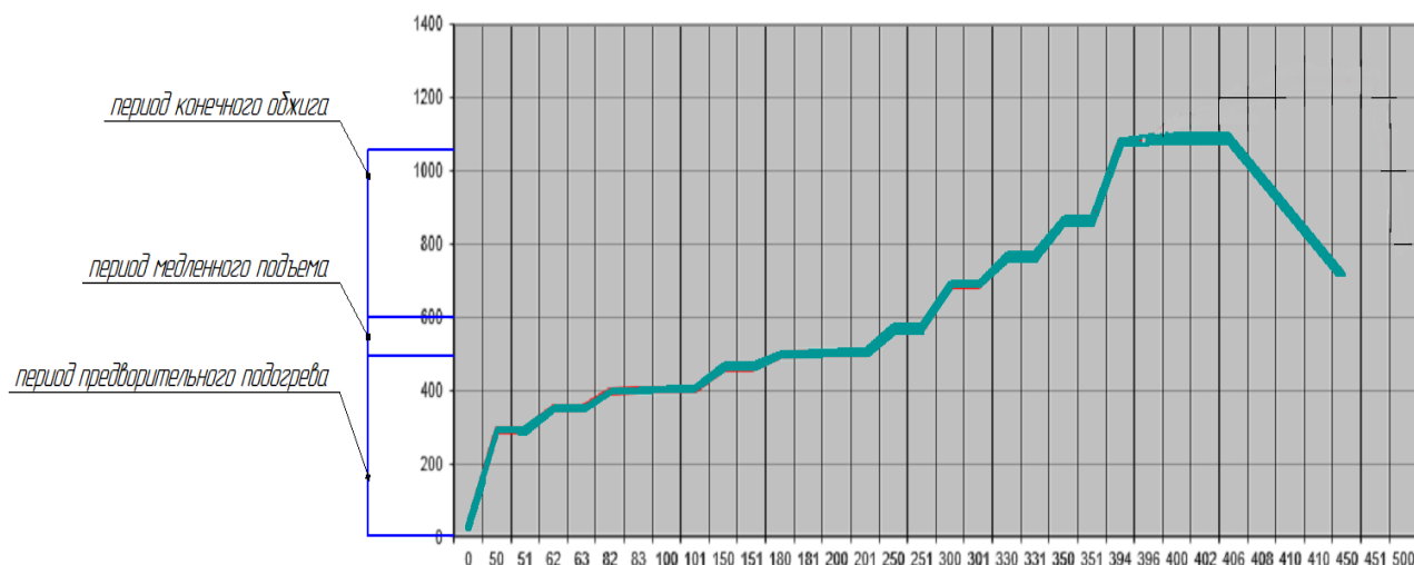
Рис. 2. Кривая изменения температуры во времени (кривая обжига)
