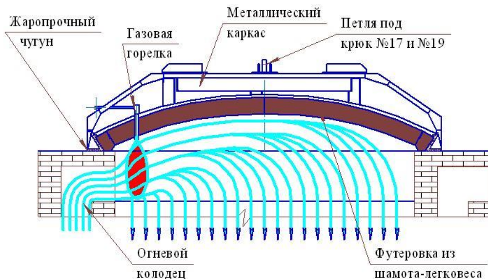
Рис. 3. Разрез подсводового пространства камеры
