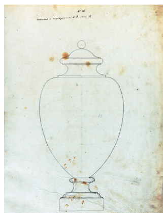
Ил. 14. Схематичное изображение яйцевидной вазы с крышкой. Перо, тушь. 498 × 362 мм. Колыванский альбом № 3. Л. 13. Государственный Эрмитаж, Санкт-Петербург, 2021. Фото Д. А. Бобровой
