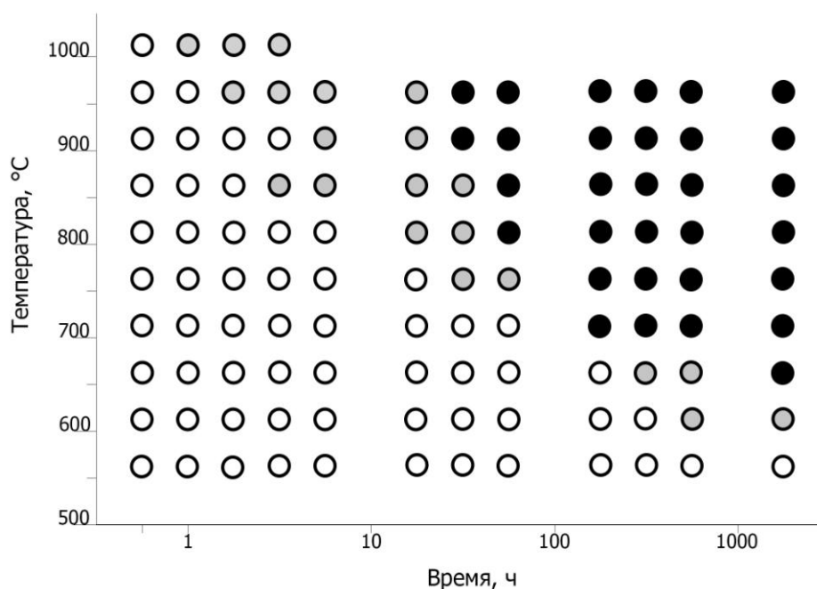
Рис. 1. Диаграмма «время – температура – фазовый состав» для модифицированного сплава ХН63МБ с пониженным содержанием углерода.
